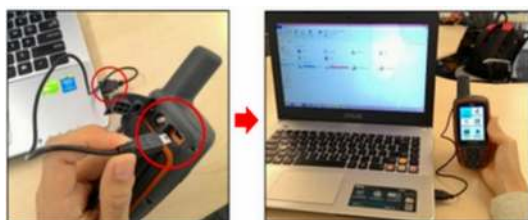
“Menyambungkan GPS dengan kabel ke Laptop”
